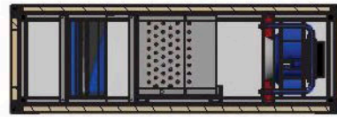
A-A (1 : 18)
